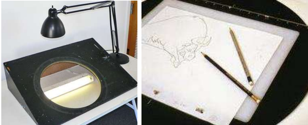
Gambar 11.2 LigthBox
