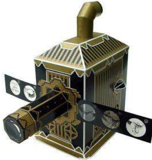
Gambar 1.5 Lentera Ajaib
