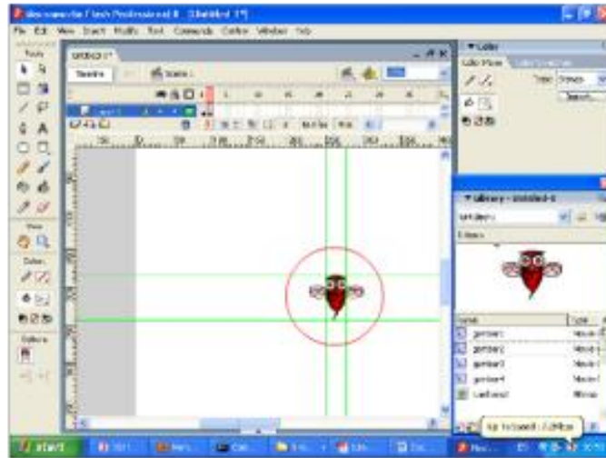
Gambar 19.20 Langkah 19
