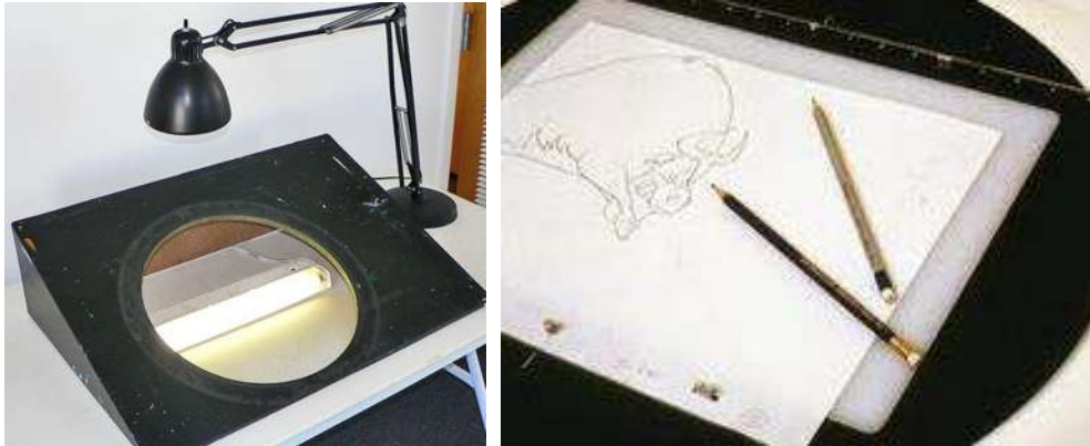
Gambar 17.2 LigthBox
