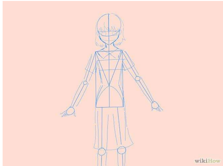
Gambar 16.9 Langkah 9
