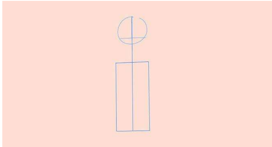
Gambar 16.2 Langkah 2
