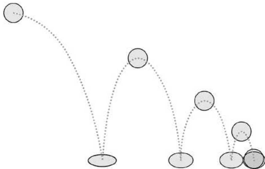
Gambar 12.4 posisi keyframe
